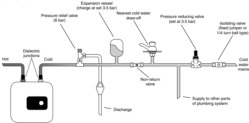
Fig. 2 Europrisma EP 10/15
